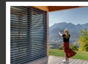
Brise-soleil orientables. Récepteur radio BiLine Combio «JA» et moteur radio confort ECB.
